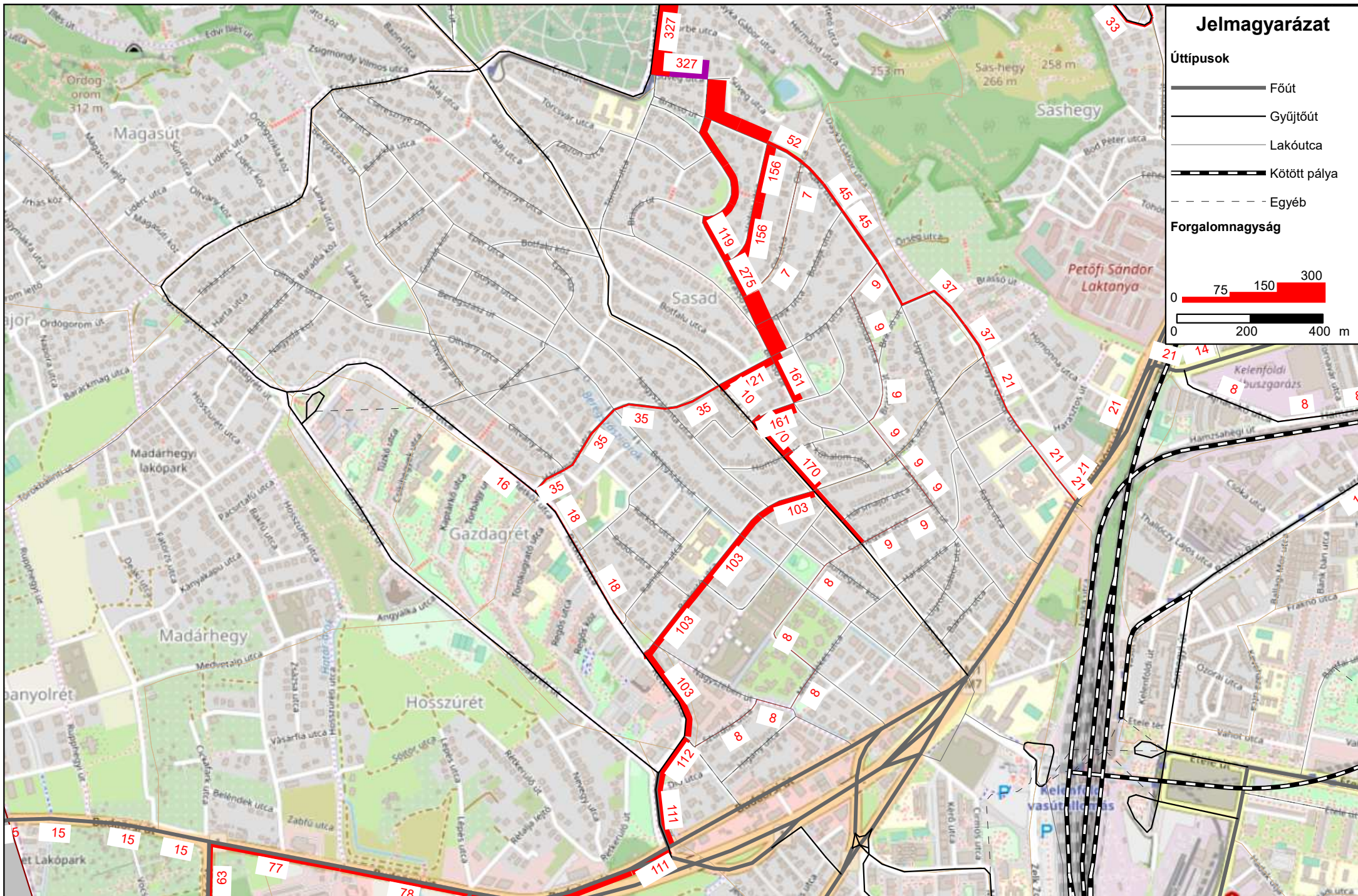
Süveg utca forgalomáramlása keletről-nyugatra [EJM/óra]
