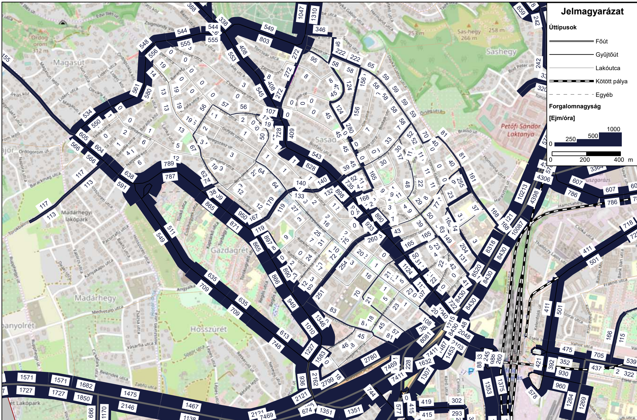
Sasad és környékének forgalomáramlási ábrája – meglévő állapot
